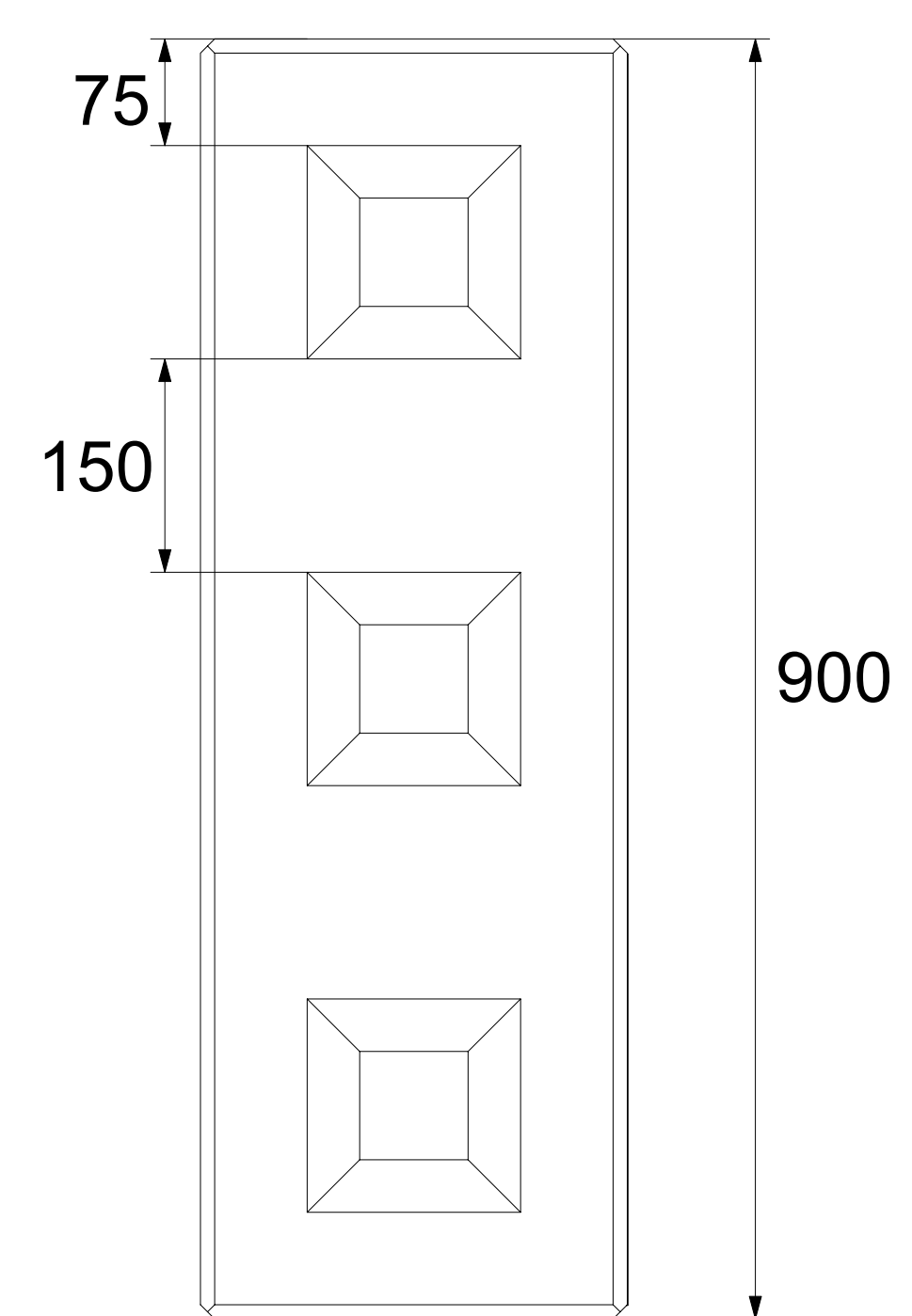
Rzut poziomy
