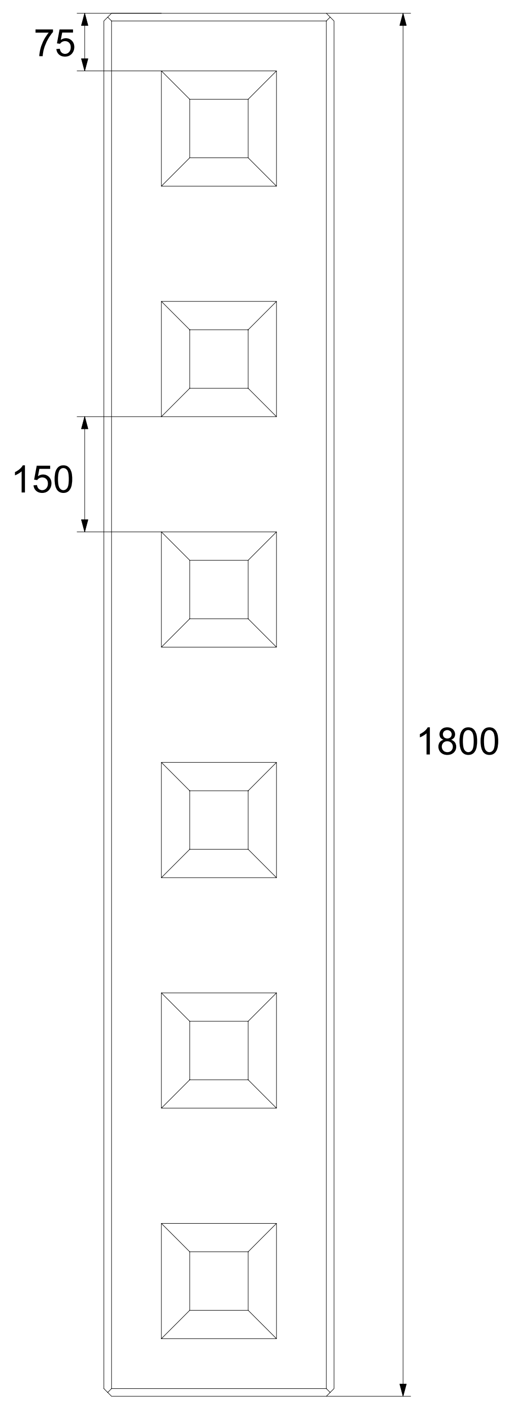
Rzut poziomy
